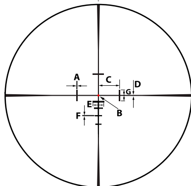
3TR/P3TR RETICLE SUBTENSION
